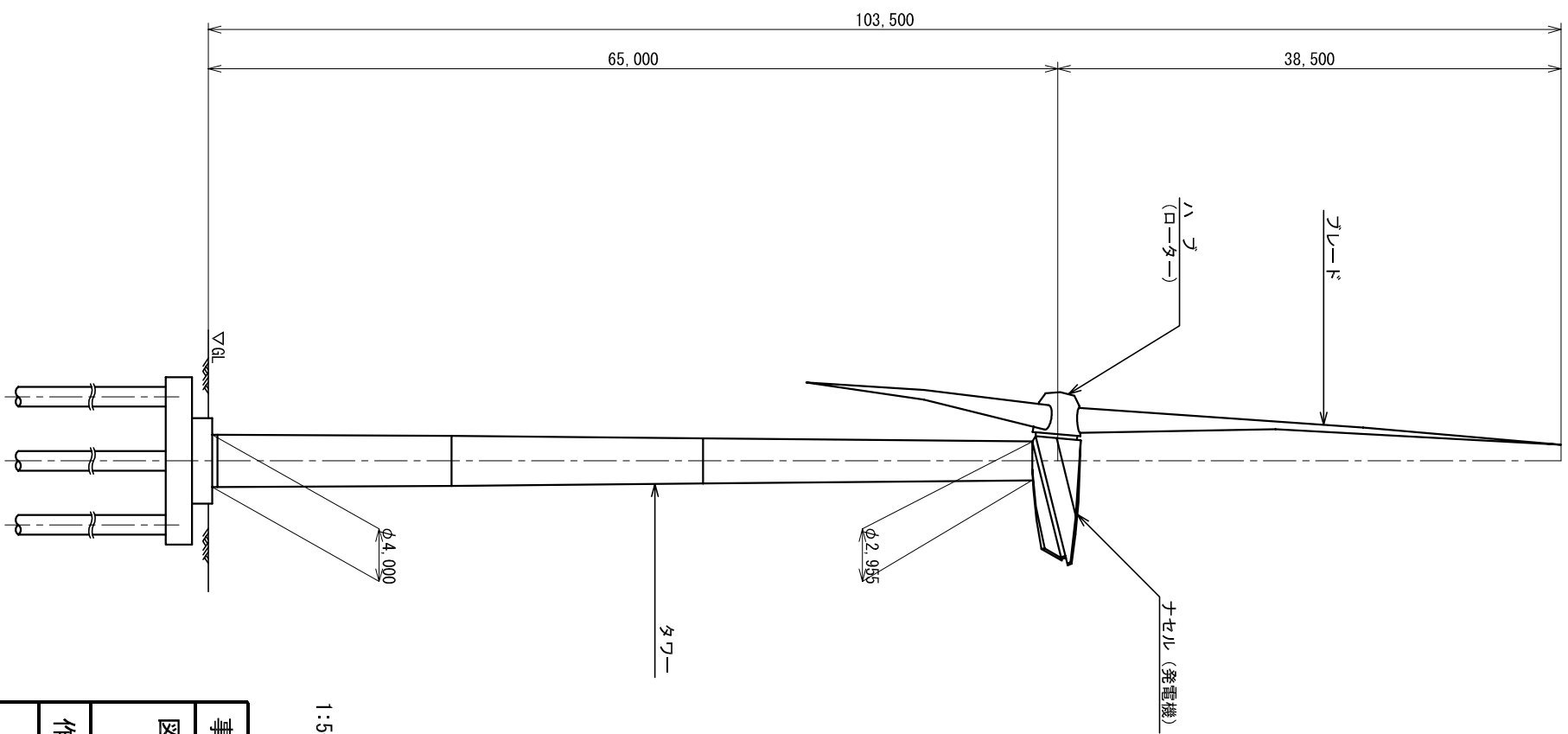
側面図
